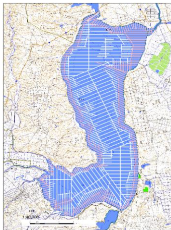
測量計画図
